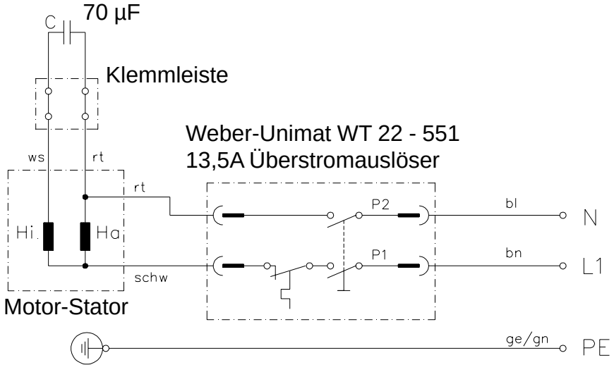
Schaltbild für KRÄNZLE 145 T 230 Volt / 50 Hz
