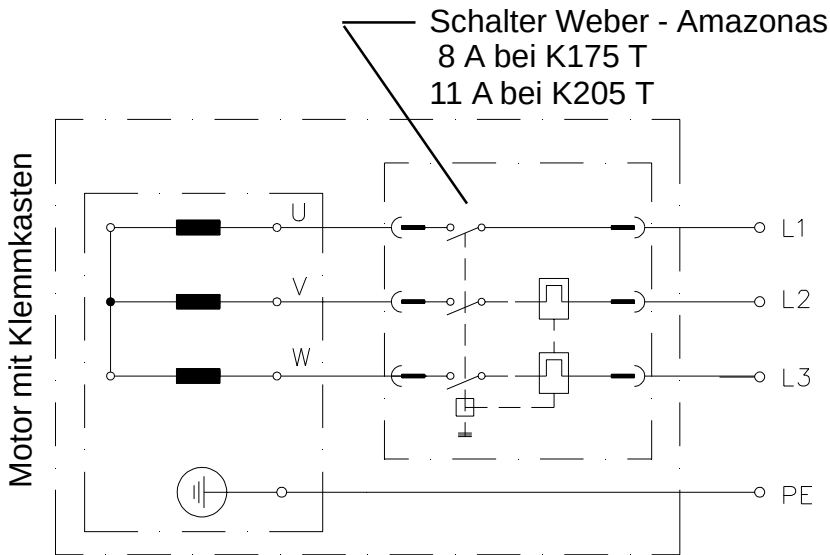
Schaltbild für KRÄNZLE 175 T und 205 T 400 Volt / 50 Hz
